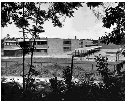
Vasemmalla: Puotilan kansakoulussa jokaisella luokka-asteella oli oma paviljonkinsa. Kuva: Simo Rista / Arkkitehtuurimuseon kuvakokoelmat. Oikealla: pohjapiirroksesta näkyy, miten koulurakennus on jäsenneilty eri luokka-asteille tarkoitettuihin paviljonkeihin. Koulun pihat ryhmittyvät vastaavasti paviljonkien ympärille. Kuva: Arkkitehtuurimuseo.
